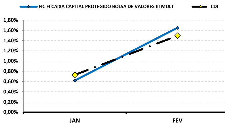
Rentabilidade Acumulada
